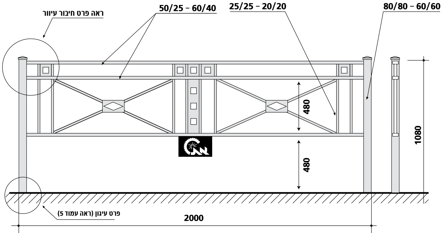
אלטרנטיבה א' (עמוד/מסגרת)
